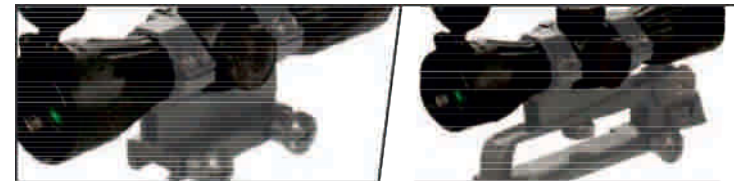
С-5. Кронштейн для установки на ствольную коробку или на ручку для переноски
